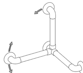
A DOS PAREDES CON 3 TRAMOS UNIDOS
